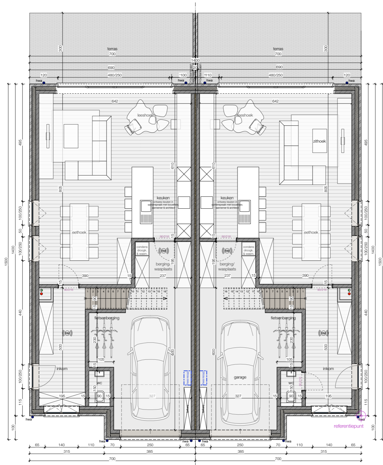
GRONDPLAN
